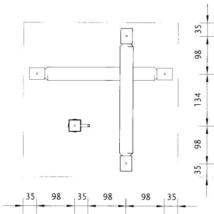
Onderaanzicht View from underneath
